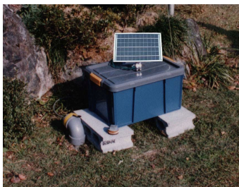
太陽電池 DC12V、8W～
